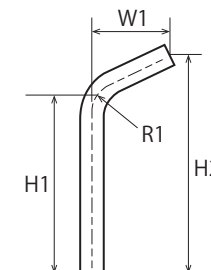
曲げパイプ (自由曲げ)
