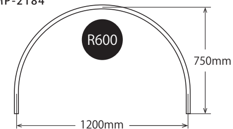
規格曲げパイプ (180度曲げ)
