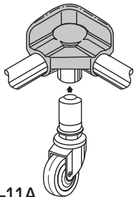
JG-11A 積み重ね受け用 別売りのキャスターをパイプに取り 付けることもできます。ジョイントに 直接キャスターを取り付けることは できません。
