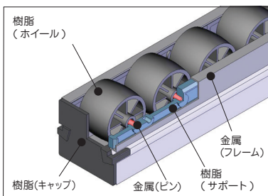
▲クリフォームプラコンの構成と材質
