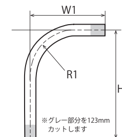
曲げパイプ (90度曲げ)
