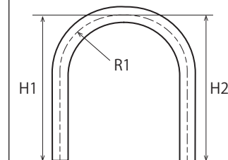
曲げパイプ (180 度曲げ)
