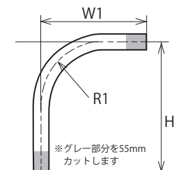
曲げパイプ (90 度曲げ)
