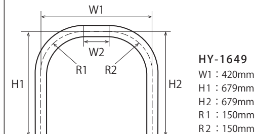
曲げパイプ (90度曲げ・2曲げ)
