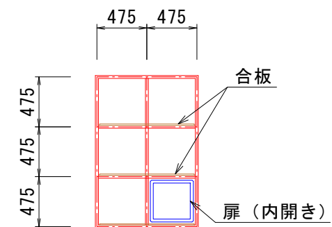
断面図②
