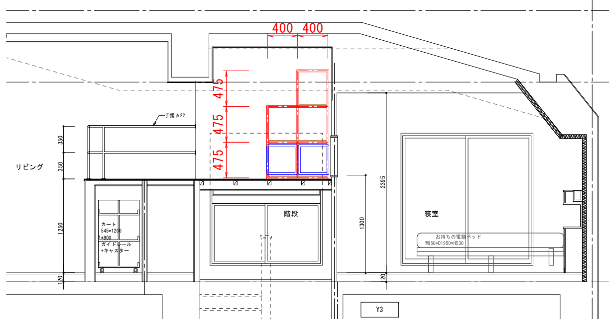
断面図①
