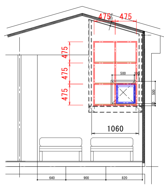
断面図②
