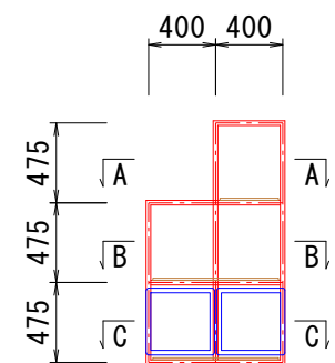
断面図①
